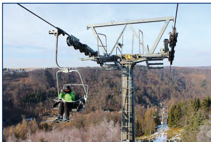
Trasa lanovky – podpěra č. 6
